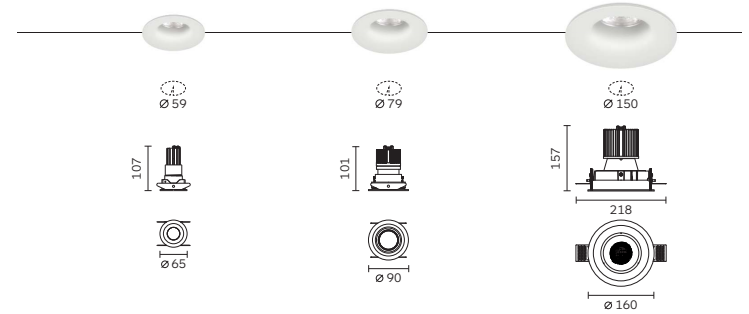
Ovo 65 / 90 / 160 Fixed Trim
