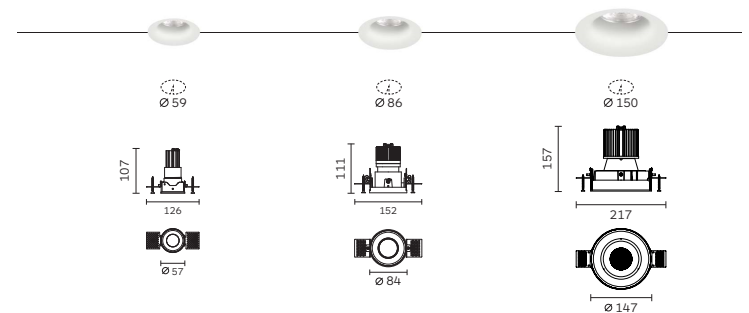
Ovo 65 / 90 / 160 Fixed Trimless
