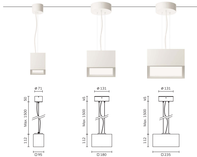
DomoLED 95 / 180 / 235 Square Pendant
